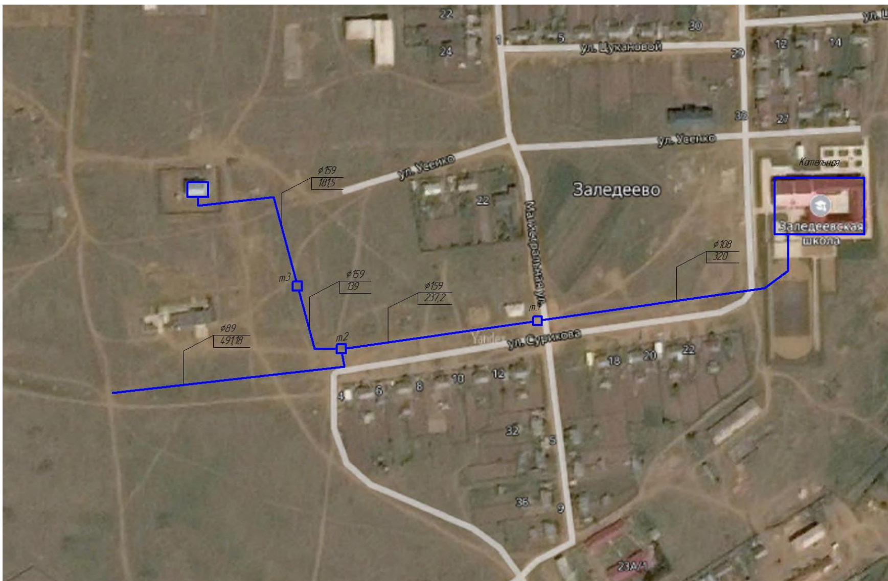
Рисунок 1.3.2.2. Принципиальная схема теплоснабжения Заледеевского сельсовета котельная «Школа»
