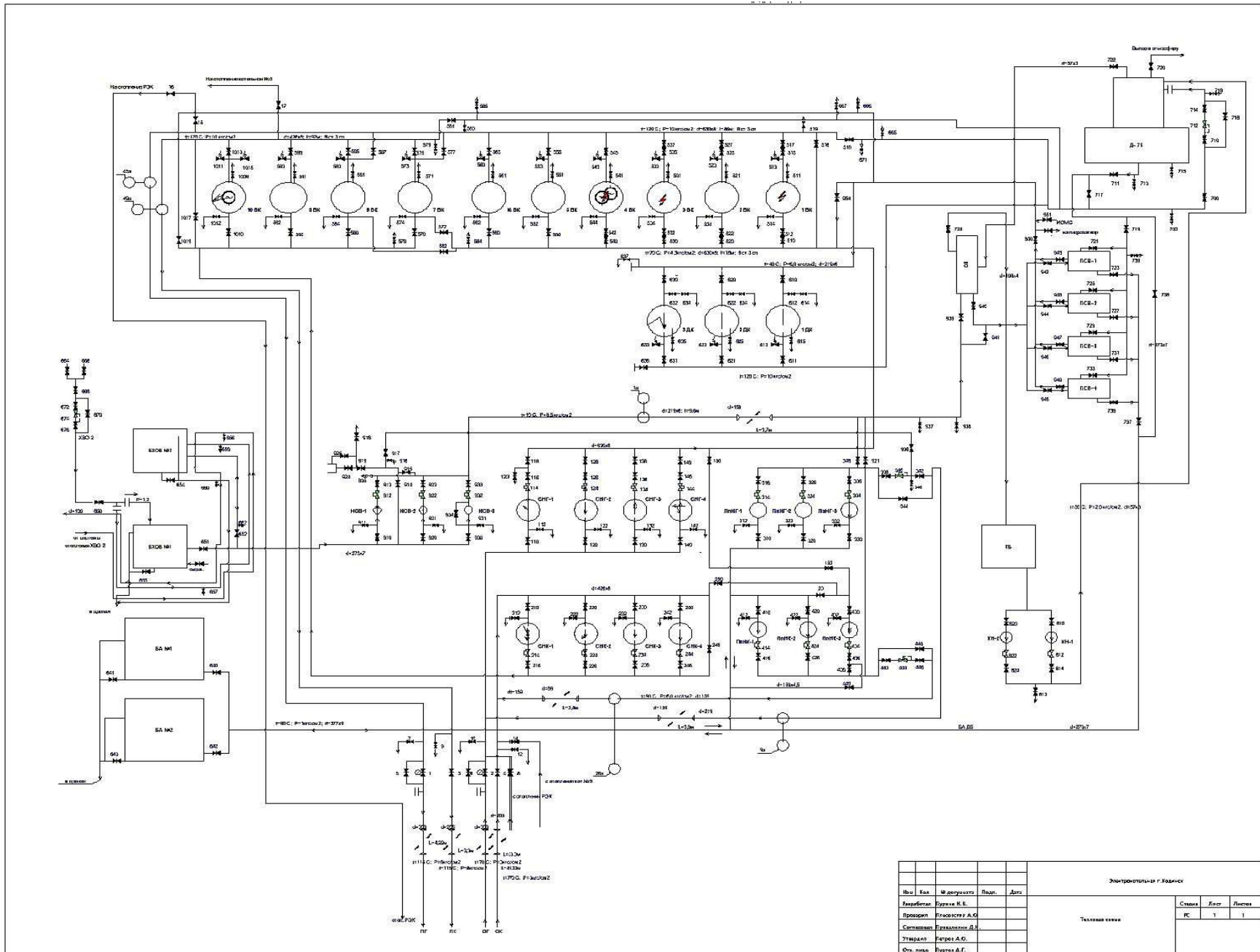
Рисунок 2.3 – Принципиальная схема котельной города Кodinginsk
