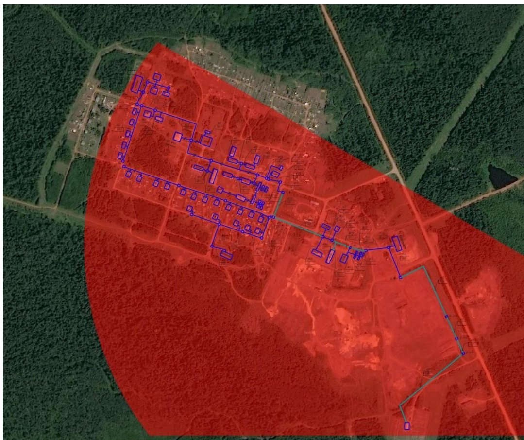
Рисунок 7.15.1. Радиус теплоснабжения котельной «Поселковая» п. Имбинский
