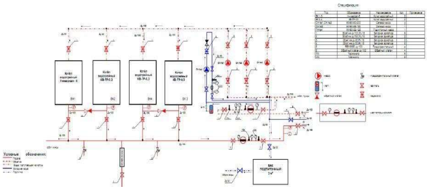
Рисунок 4. Технологическая схема котельной №2 п. Недокура
