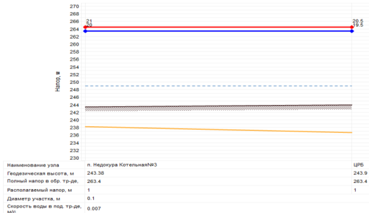
Рисунок 10. Пьезометрический график от котельной № 3 до потребителя «ЦРБ»
