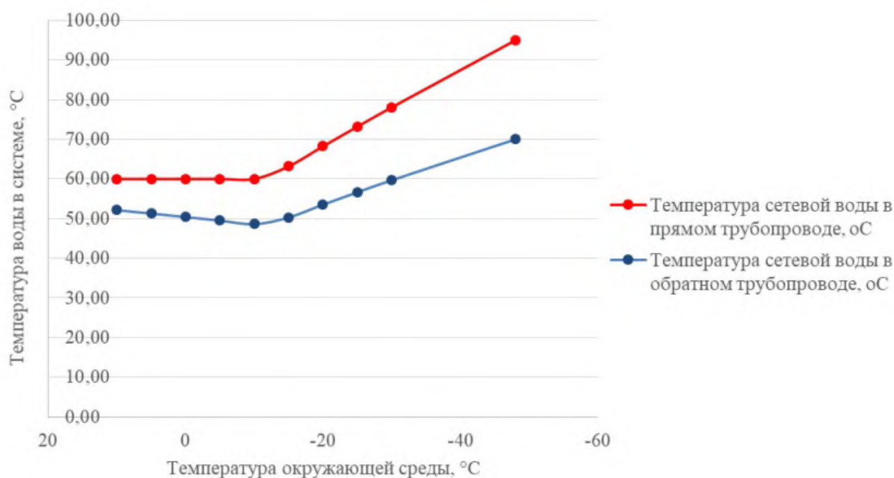
Рисунок 2.4 – График изменения температур теплоносителя (температурный график 95/68^{\circ}\text{C} )
