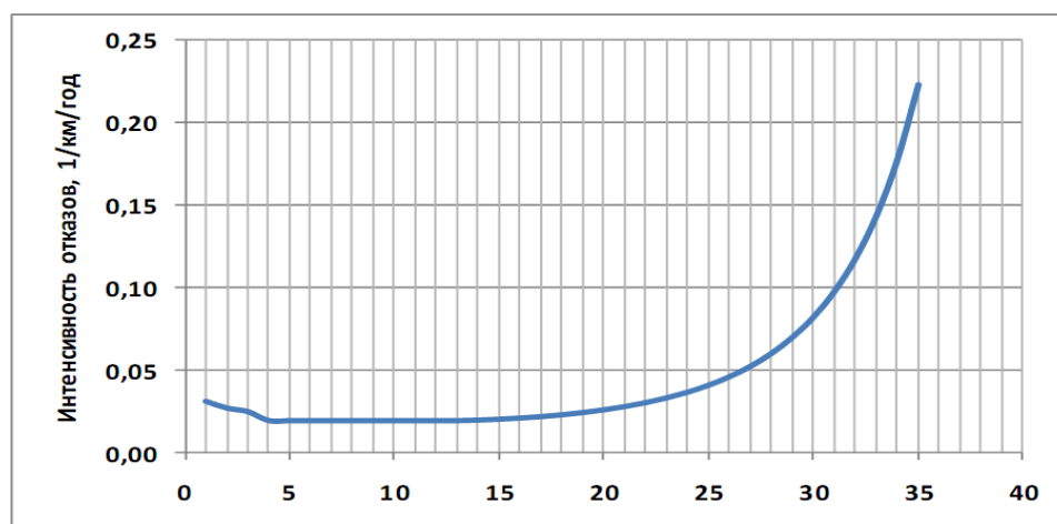
Рисунок 12. Интенсивность отказов в зависимости от срока эксплуатации участка тепловой сети
