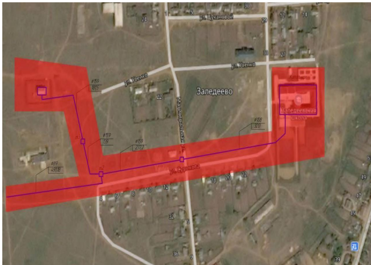
Рисунок 9. Зона действия источника теплоснабжения котельная «Школа»
