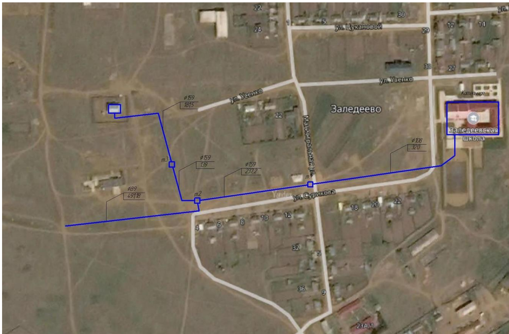
Рисунок 5. Принципиальная схема теплоснабжения Заледеевского сельсовета, котельная «Школа»
