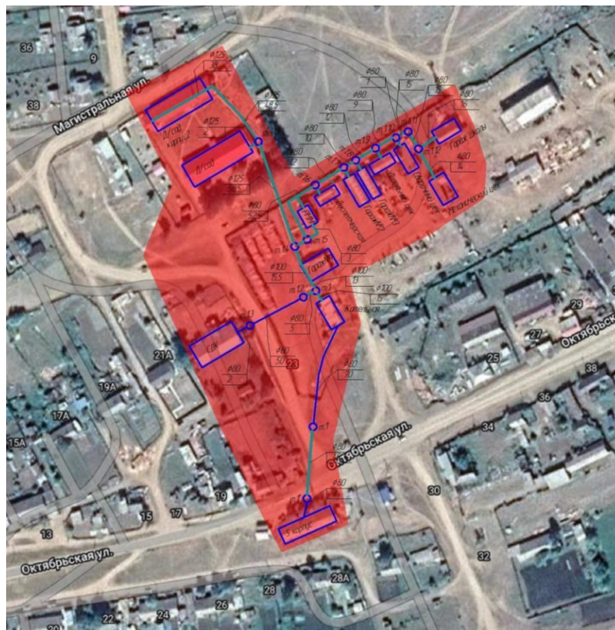
Рисунок 8. Зона действия источника теплоснабжения котельная «Поселковая»
