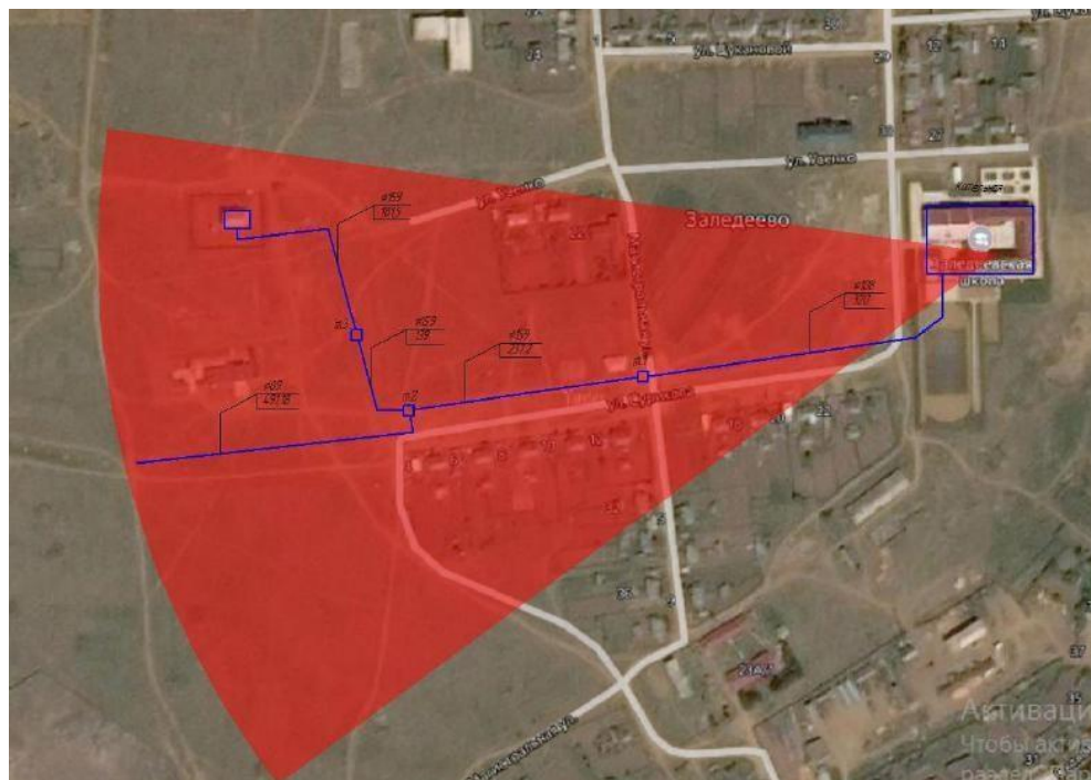
Рисунок 11. Радиус теплоснабжения котельной «Школа» с. Заледеево
