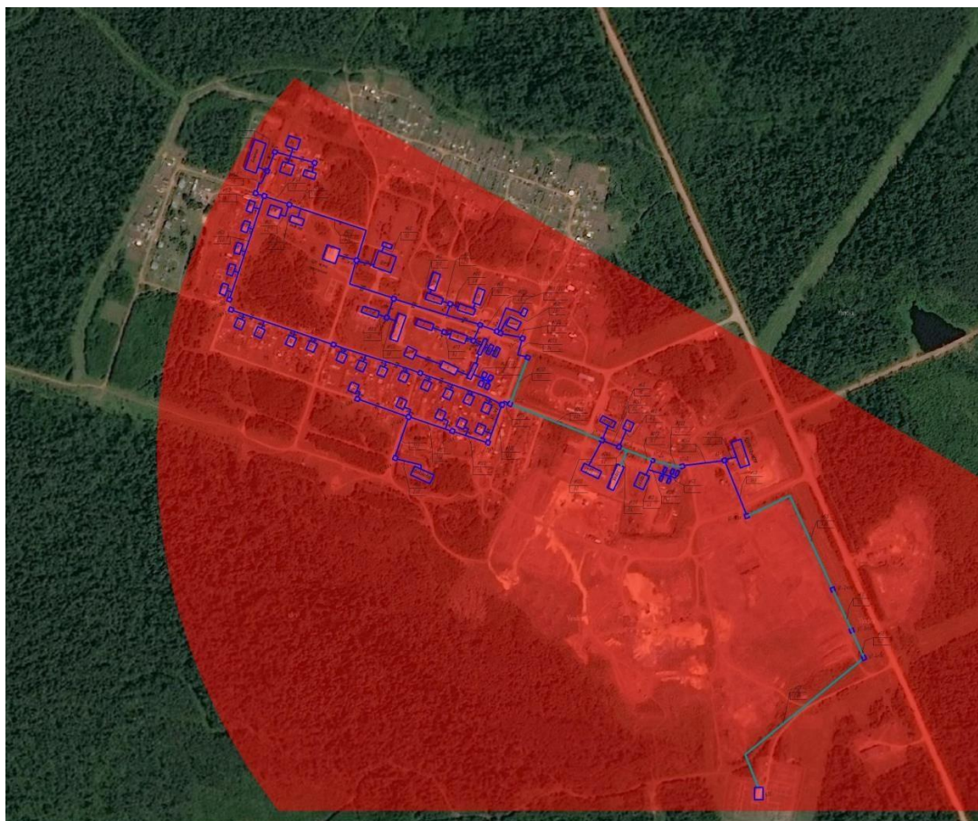
Рисунок 8. Радиус теплоснабжения котельной «Поселковая» п. Имбинский
