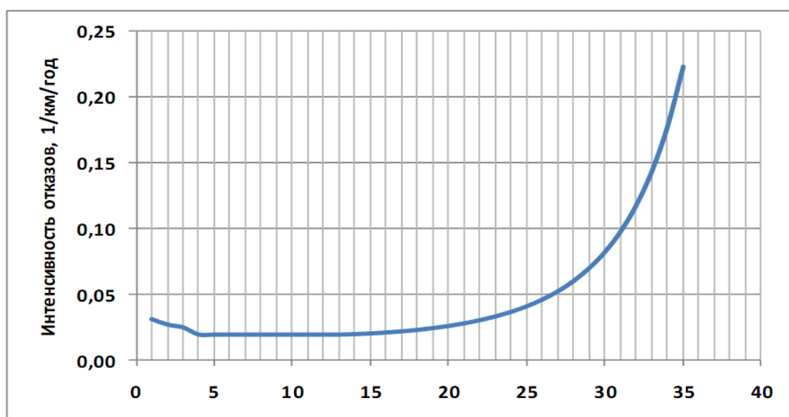
Рисунок 9. Интенсивность отказов в зависимости от срока эксплуатации участка тепловой сети
