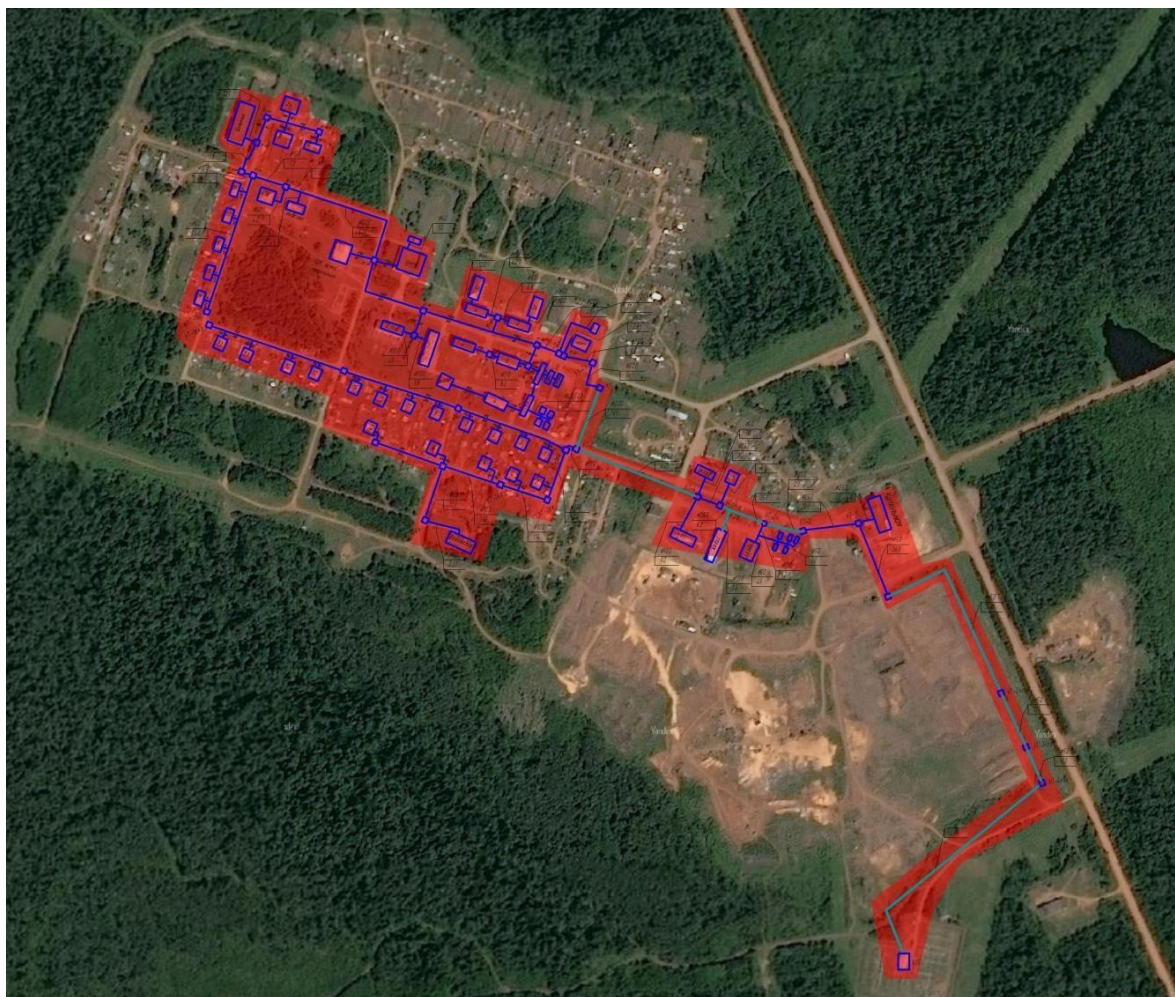
Рисунок 7. Зона действия источника теплоснабжения котельная «Поселковая»
